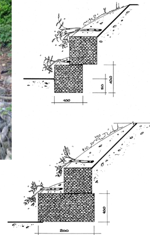
GABBIONATA CON TALEE
